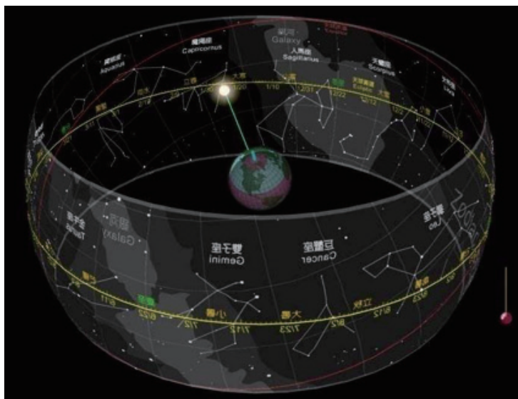
图3. 黄道带
