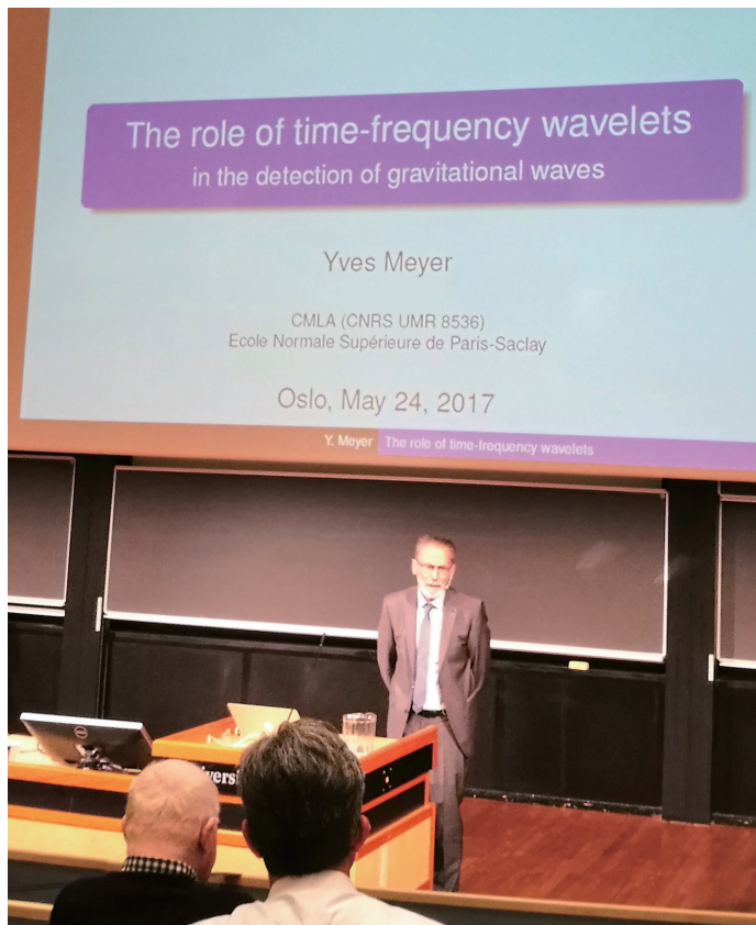
接受阿贝尔奖后的学术演讲：“时域小波在引力波观测中的作用”
