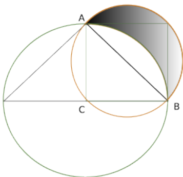
阴影部分弓月形的面积等于直角三角形ABC的面积
