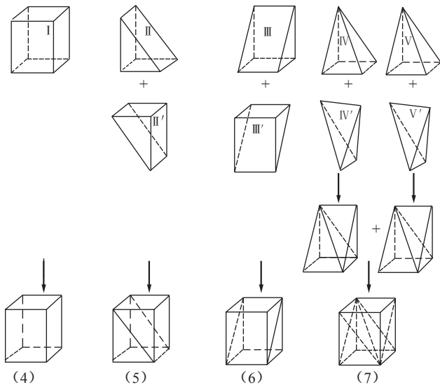
图9 刘徽原理之证明
