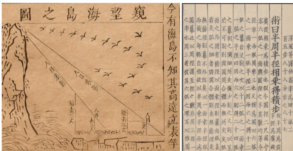
图4 刘徽测望海岛示意图
