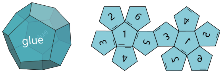
左图展现了正十二面体一组对面的粘合方式，其余五组对面粘合的规则类似。右图是正十二面体的外表面展开图，完整标记了各组对面的粘合方式。
